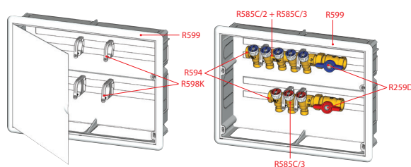
Установка в шаф R599
